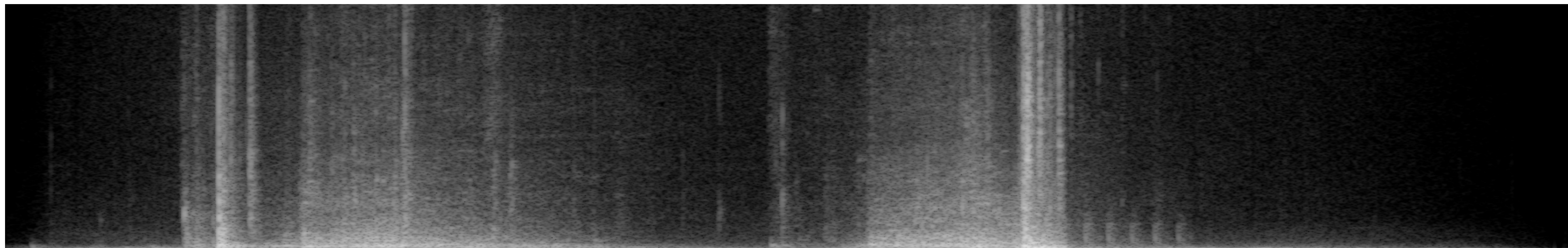
Звукова спектрограма: Зачиняються двері буса (див. стор. 17)
