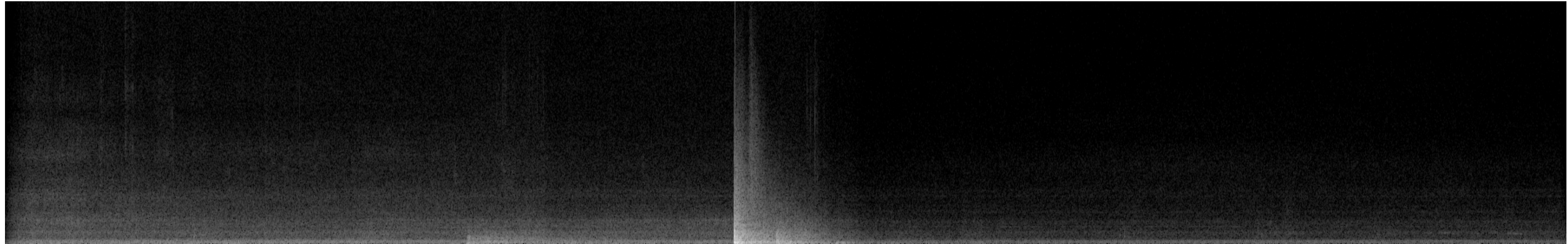
Звукова спектрограма: Вибухи
