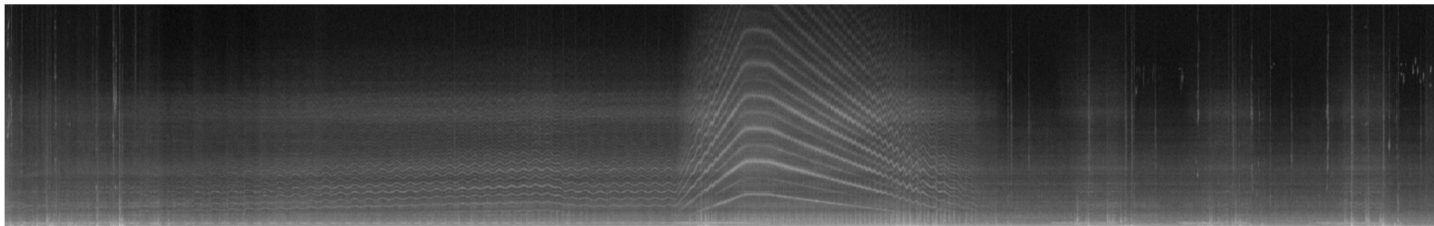
Звукова спектрограма: Барабани пральної машини (див. стор. 14)
