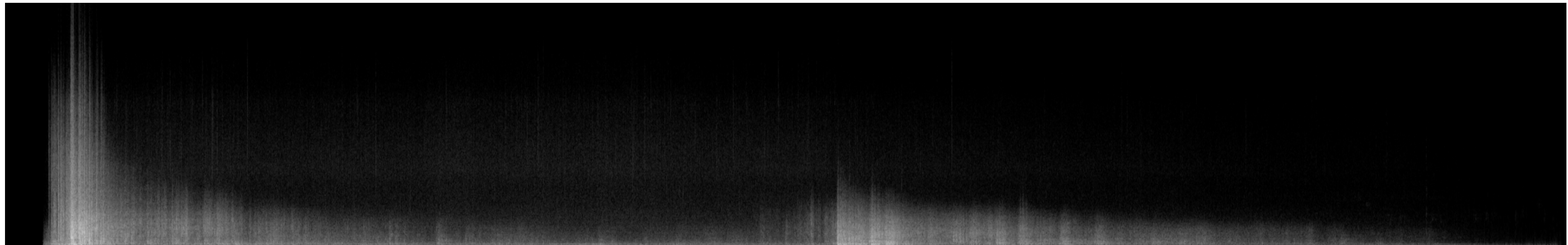
Звукова спектрограма: Грім
